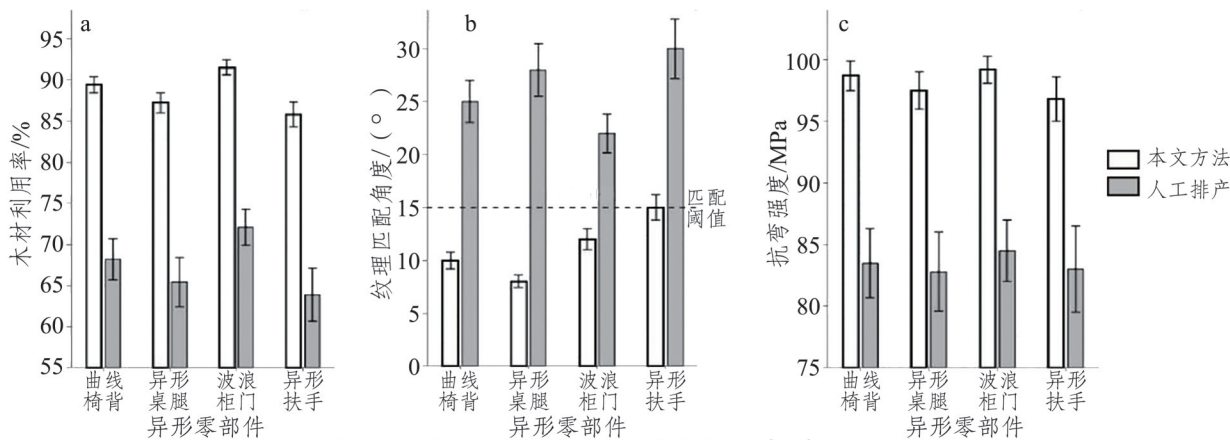
图9 异形零部件排料性能对比:改进遗传算法 vs. 人工排料
