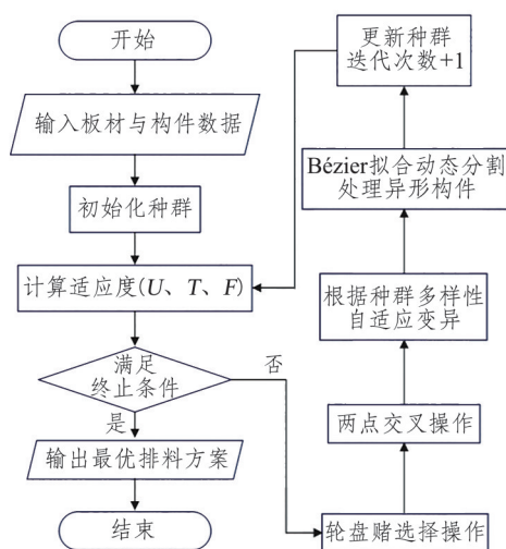
图5 改进遗传算法的流程
