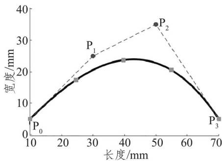
图6 Bézier曲线动态分割示意
