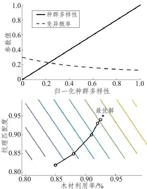
图7 自适应变异策略(变异概率与多样性关系)与解空间搜索过程示意
